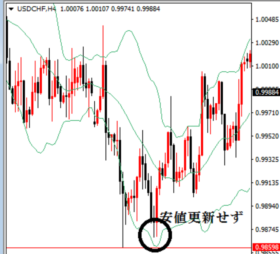
USDCHF,H4
